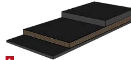
1 Die Abbildung zeigt den Aufbau eines germanBelt-Textilfördergurtes
